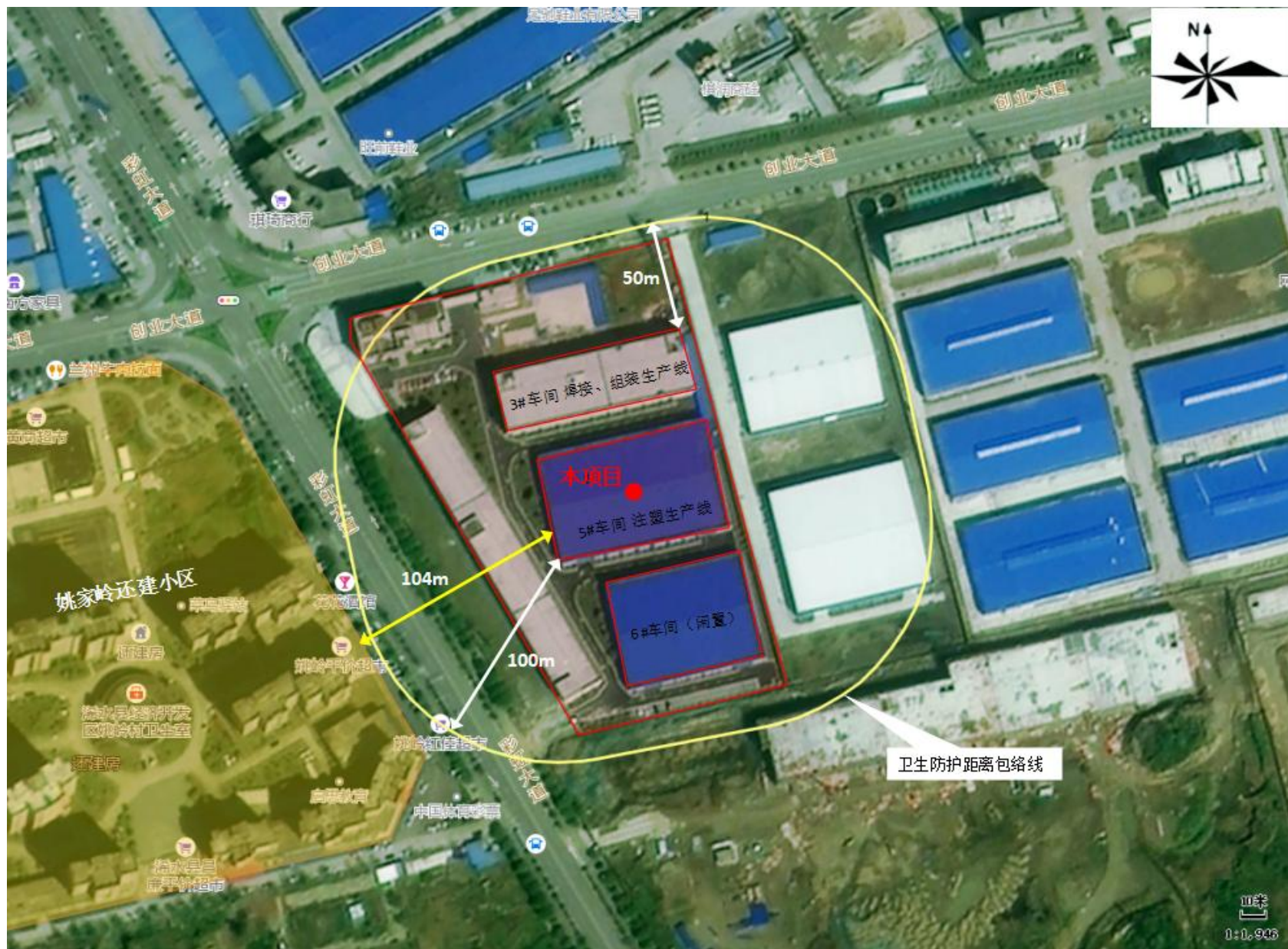
附图 5 项目卫生防护距离包络线图
